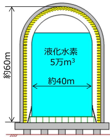
5万m 3 液化水素貯槽
