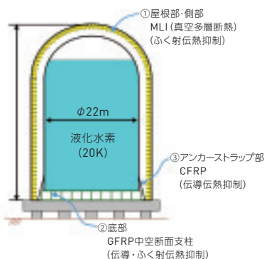
図 液化水素タンク断熱構造
